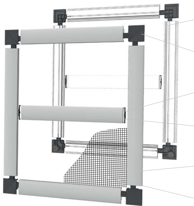
PERFIL CURVO
